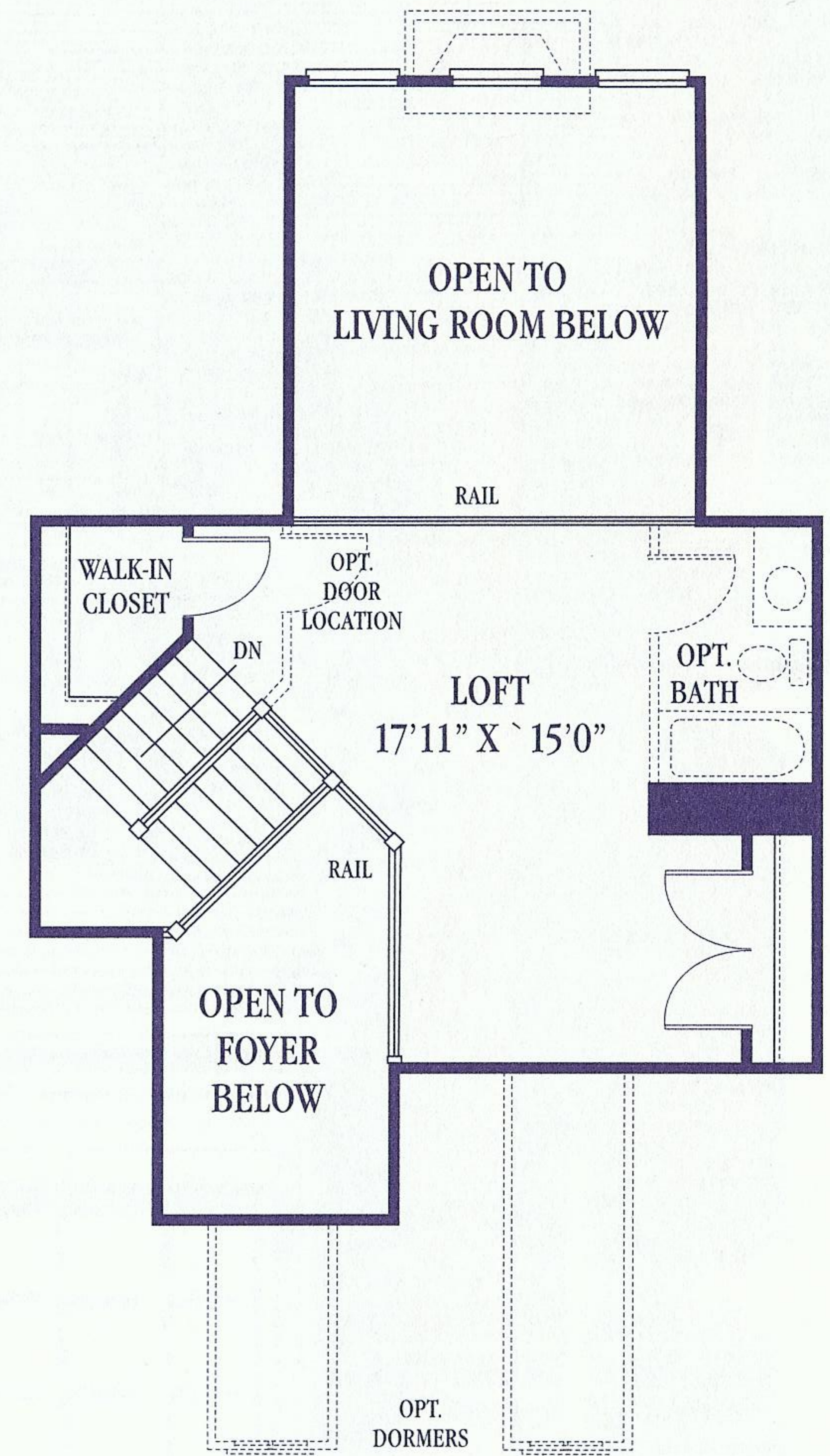
OPTIONAL LOFT
